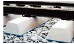
まくらぎパッド Under Sleeper Pads
