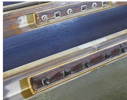
接着絶縁レール (JIS) Glued Insulated Rails
