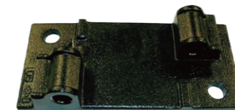
パンドロール用 (鋳造タイププレート) For Pandrol Fastening (Cast Tie Plate)
