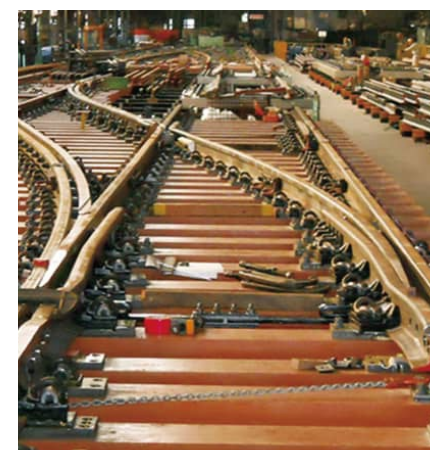
渡り線(レール製、5# R=45m) Crossover (Rail Type, 5# R=45m)
