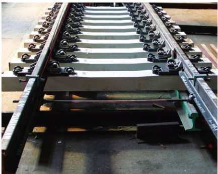
伸縮継目 (PCまくらぎ用、パンドロール式) Expansion Joint (for PC Sleepers, Pandrol Type)
