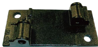
パンドロール用 (鋳造タイプレート) For Pandrol Fastening (Cast Tie Plate)
